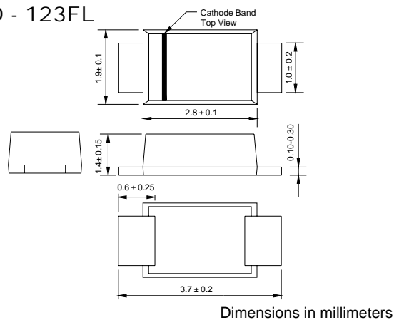
SOD - 123FL
