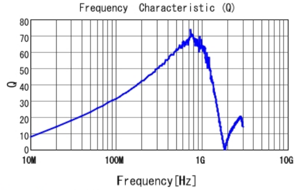
LQW18ANR15J00 Q
