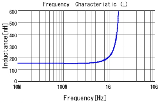
LQW18ANR15J00 L
