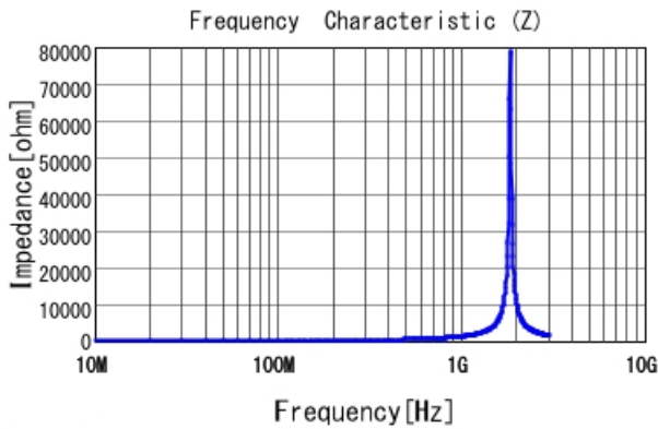
LQW18ANR15J00 |Z|
