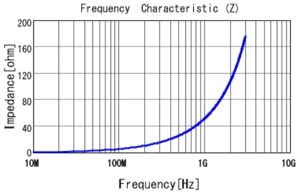
LQW18AN8N2C00 |Z|
