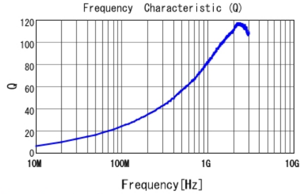
LQW18AN8N2C00 Q
