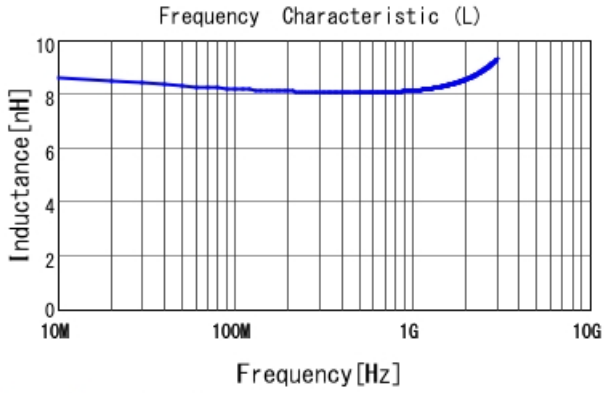
LQW18AN8N2C00 L
