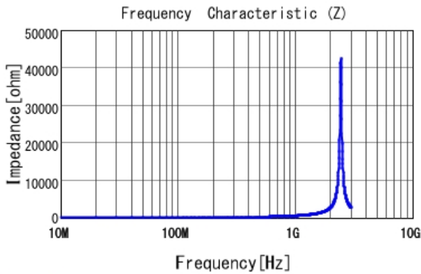
LQW18AN75NJ00 |Z|
