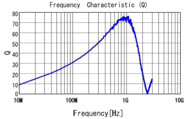
LQW18AN75NJ00 Q
