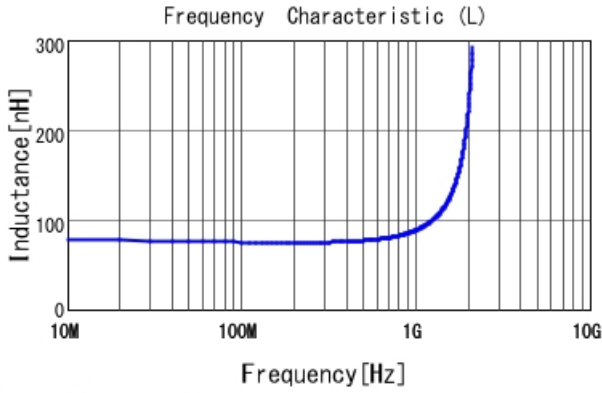
LQW18AN75NJ00 L
