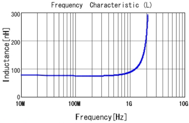
LQW18AN75NG00 L
