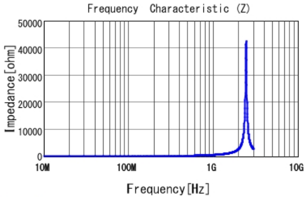
LQW18AN75NG00 |Z|
