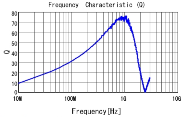
LQW18AN75NG00 Q
