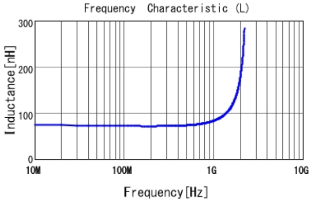
LQW18AN72NJ00 L
