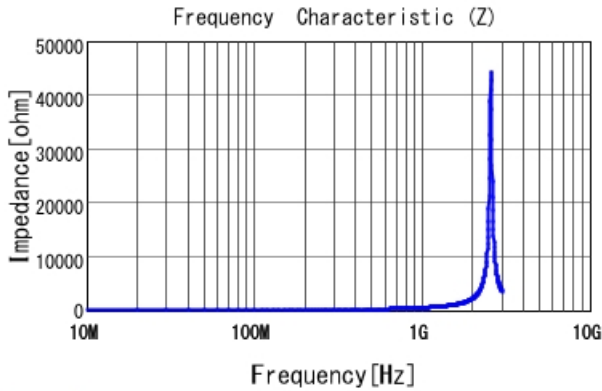
LQW18AN72NJ00 |Z|
