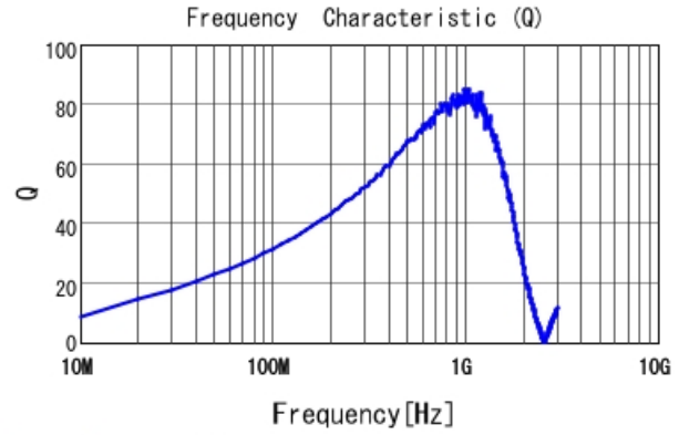
LQW18AN72NJ00 Q
