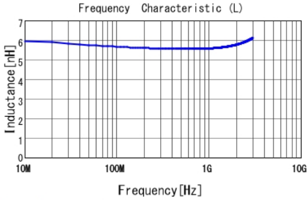
LQW18AN5N6C00 L
