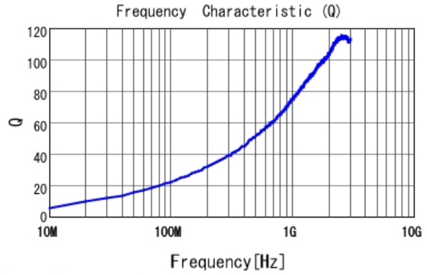
LQW18AN5N6C00 Q
