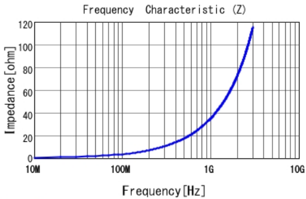
LQW18AN5N6C00 |Z|
