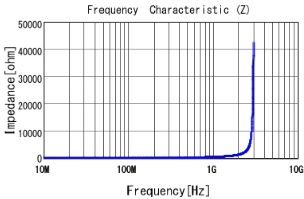
LQW18AN56NJ00 |Z|
