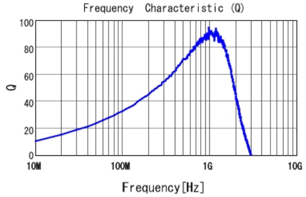
LQW18AN56NJ00 Q
