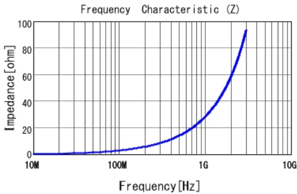
LQW18AN4N7D00 |Z|
