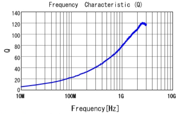
LQW18AN4N7D00 Q
