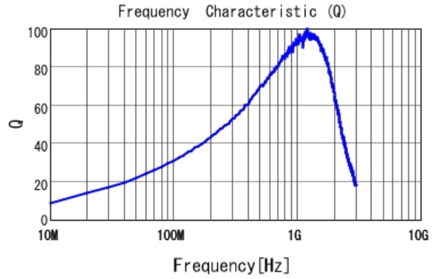
LQW18AN36NG00 Q
