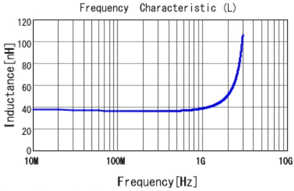
LQW18AN36NG00 L
