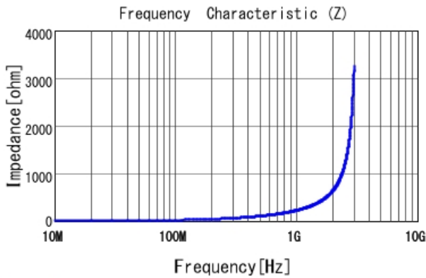
LQW18AN33NJ00 |Z|
