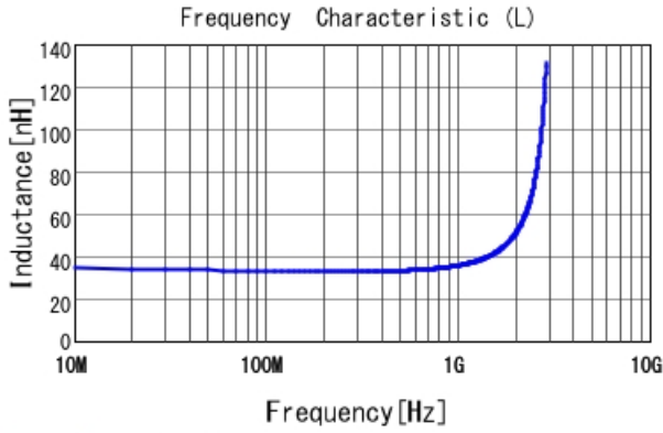
LQW18AN33NJ00 L
