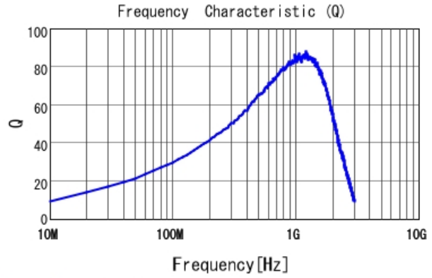
LQW18AN33NJ00 Q
