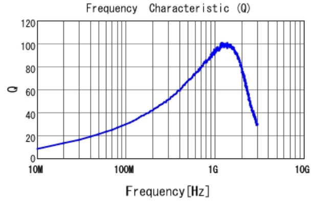
LQW18AN30NG00 Q
