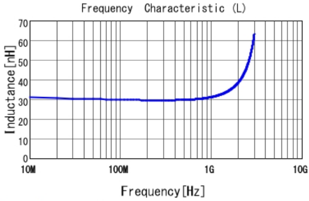
LQW18AN30NG00 L
