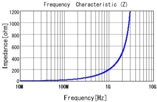
LQW18AN30NG00 |Z|
