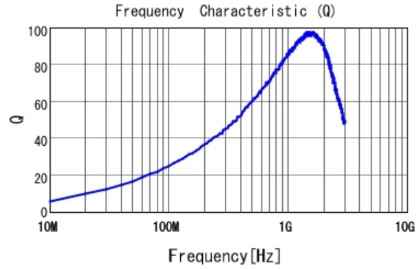
LQW18AN18NG00 Q
