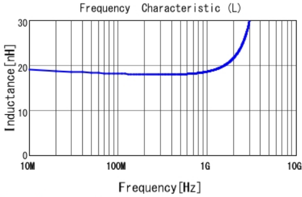
LQW18AN18NG00 L
