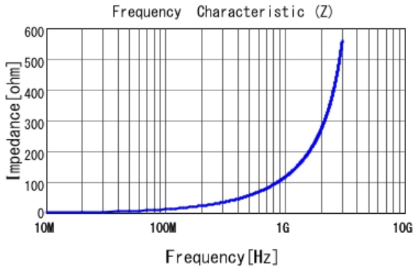
LQW18AN18NG00 |Z|
