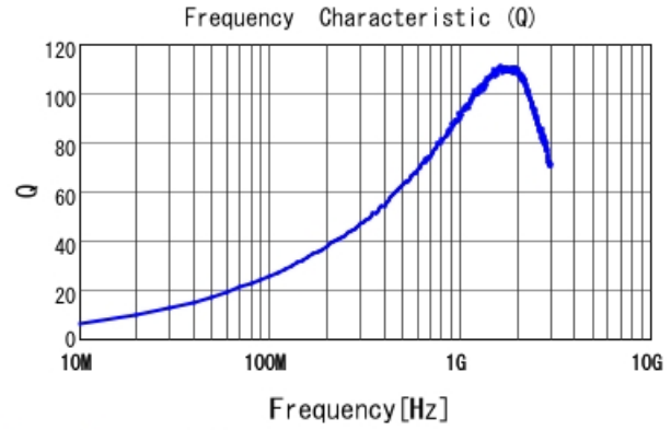
LQW18AN16NG00 Q
