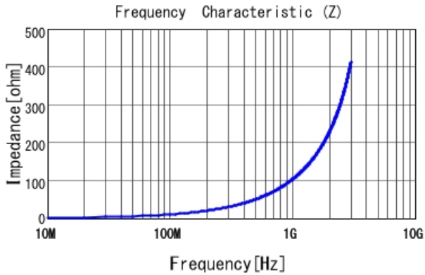
LQW18AN16NG00 |Z|
