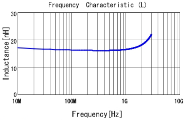
LQW18AN16NG00 L
