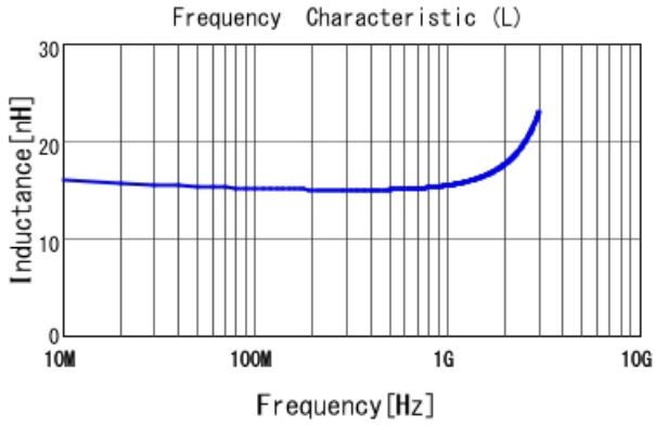
LQW18AN15NG00 L
