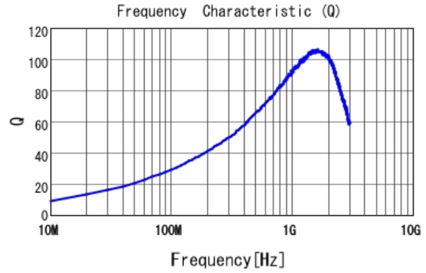
LQW18AN15NG00 Q
