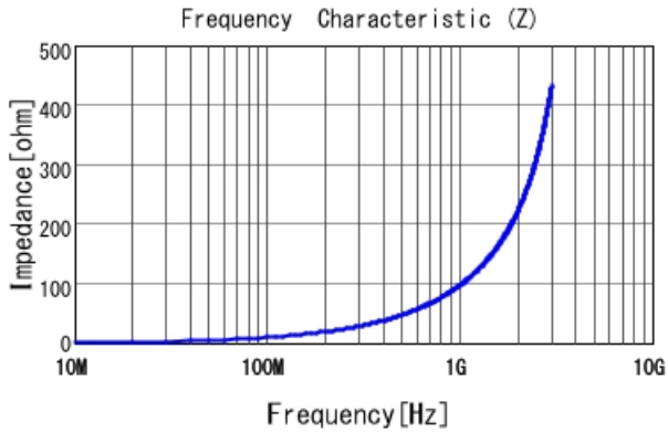
LQW18AN15NG00 |Z|
