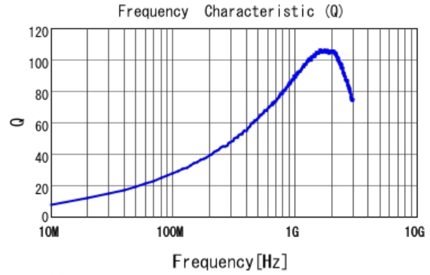
LQW18AN11NJ00 Q
