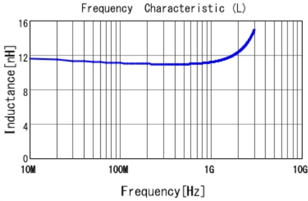
LQW18AN11NJ00 L
