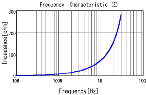
LQW18AN11NJ00 |Z|
