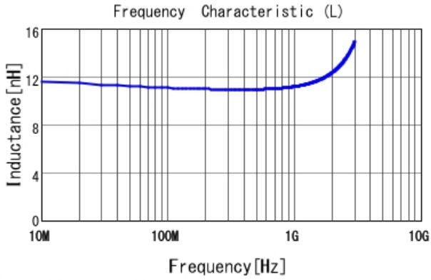
LQW18AN11NG00 L
