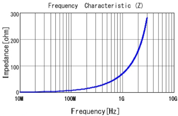
LQW18AN11NG00 |Z|
