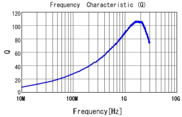
LQW18AN11NG00 Q
