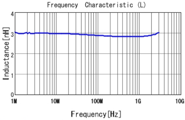
LQW15AN4N5D80 L
