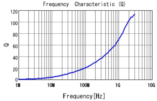
LQW15AN4N5D80 Q
