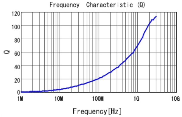
LQW15AN4N5B80 Q
