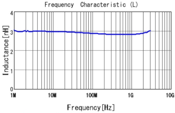
LQW15AN4N5B80 L
