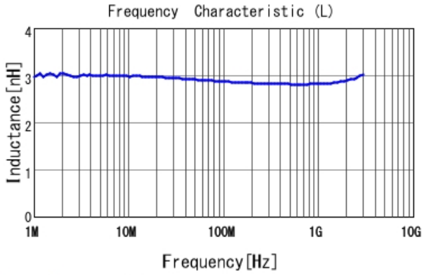
LQW15AN4N4G80 L
