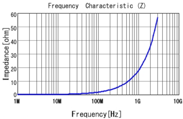
LQW15AN4N4G80 |Z|
