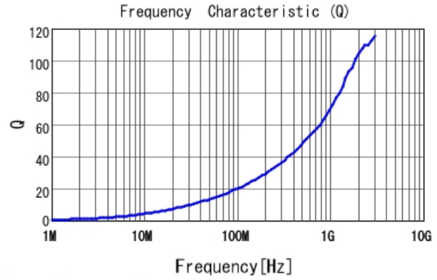
LQW15AN4N4G80 Q
