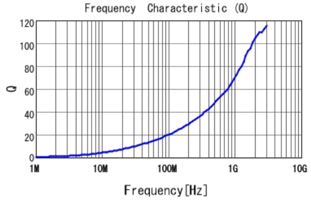
LQW15AN4N4D80 Q
