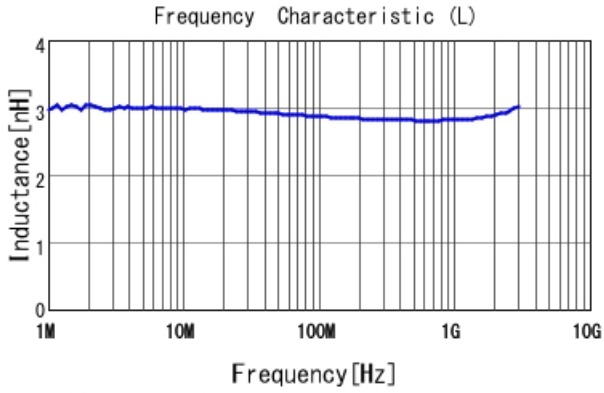
LQW15AN4N4D80 L
