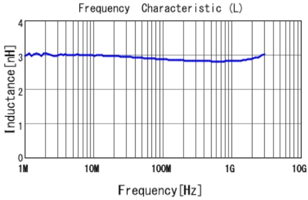
LQW15AN4N4C80 L
