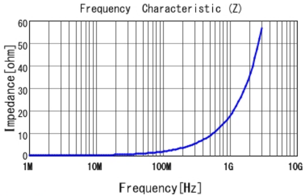
LQW15AN4N4C80 |Z|
