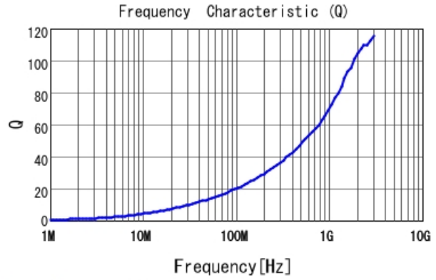
LQW15AN4N4C80 Q
