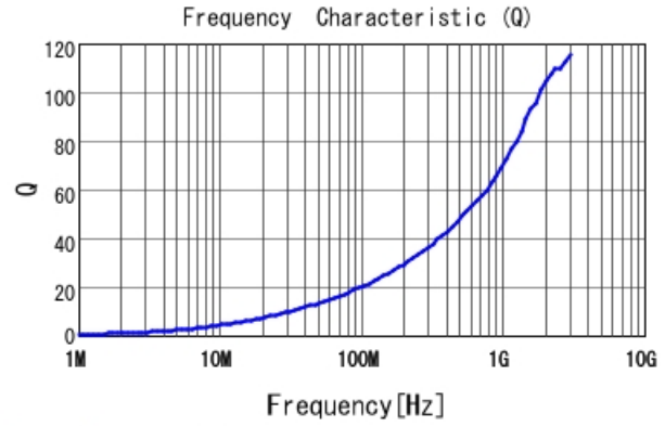
LQW15AN4N4B80 Q
