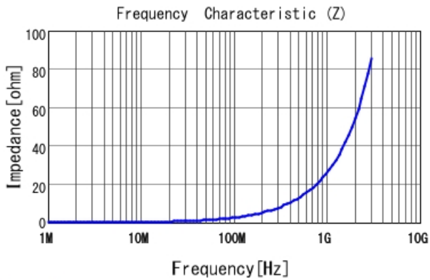
LQW15AN4N3D80 |Z|
