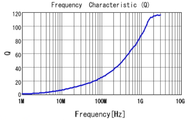
LQW15AN4N3D80 Q
