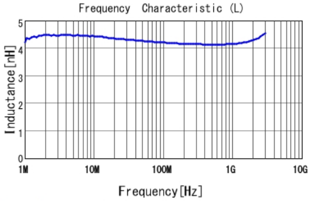
LQW15AN4N3D80 L
