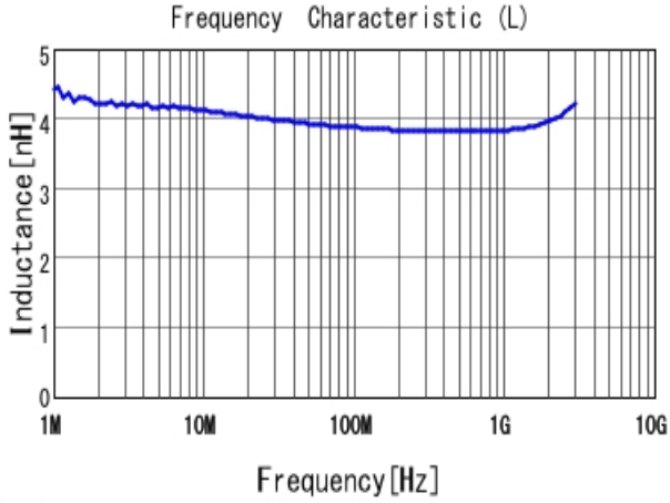
■ LQW15AN3N9G80 L
