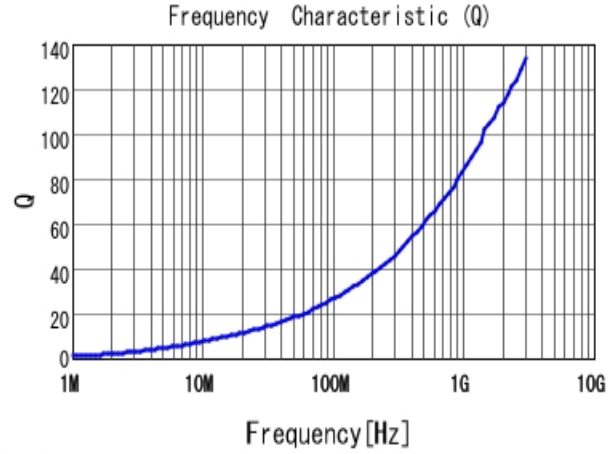
■ LQW15AN3N9G80 Q
