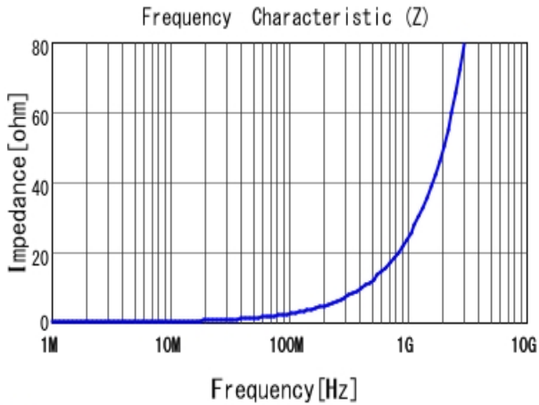
■ LQW15AN3N9G80 |Z|
