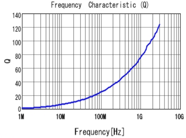
■ LQW15AN3N8G80 Q
