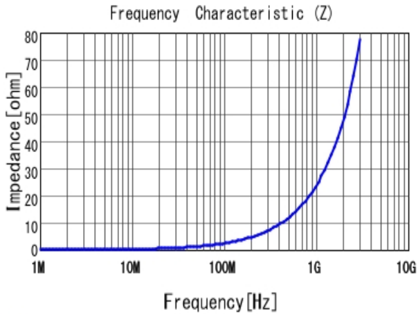
■ LQW15AN3N8G80 |Z|
