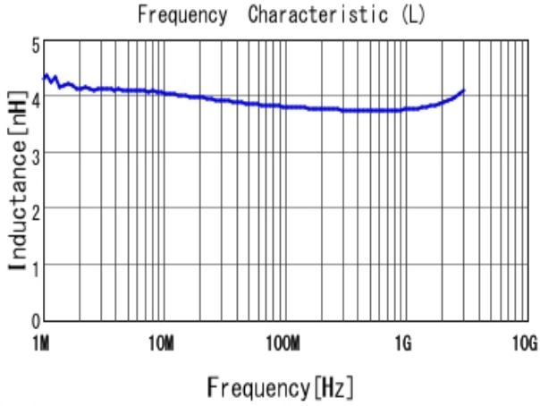
■ LQW15AN3N8G80 L
