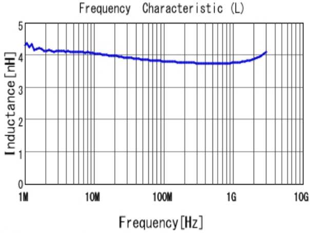
■ LQW15AN3N8D80 L
