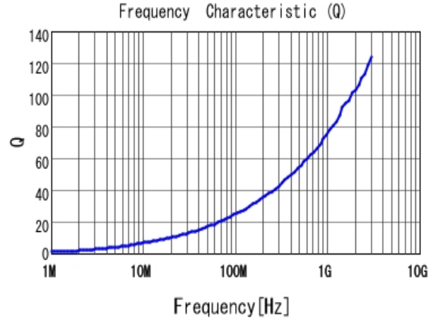
■ LQW15AN3N8D80 Q
