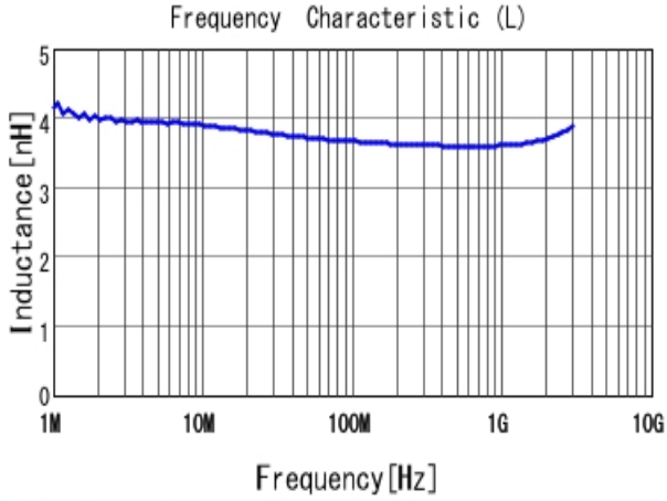
■ LQW15AN3N6D80 L
