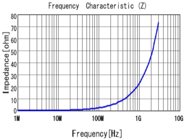
■ LQW15AN3N6D80 |Z|
