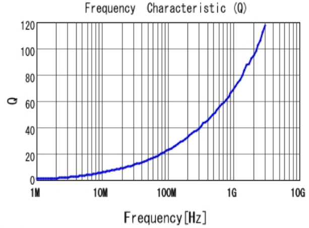
■ LQW15AN3N6D80 Q
