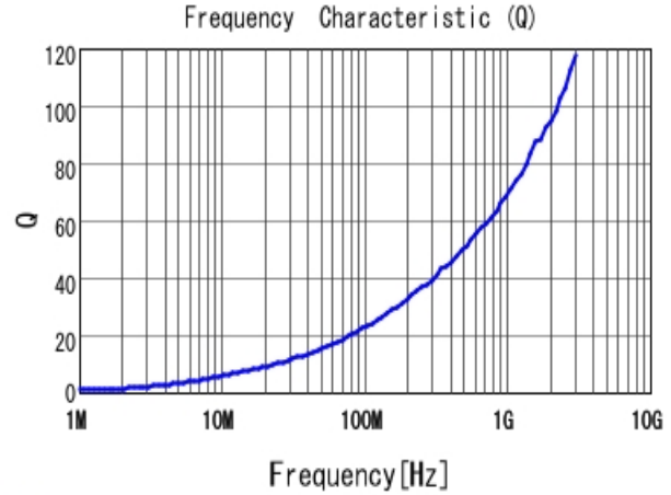
■ LQW15AN3N6C80 Q
