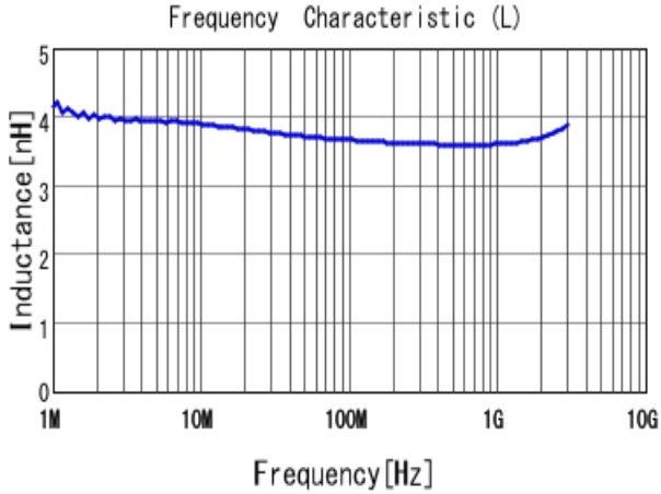
■ LQW15AN3N6C80 L
