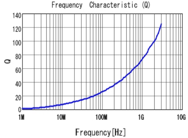
■ LQW15AN3N4G80 Q
