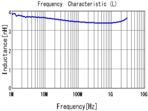
■ LQW15AN3N4G80 L
