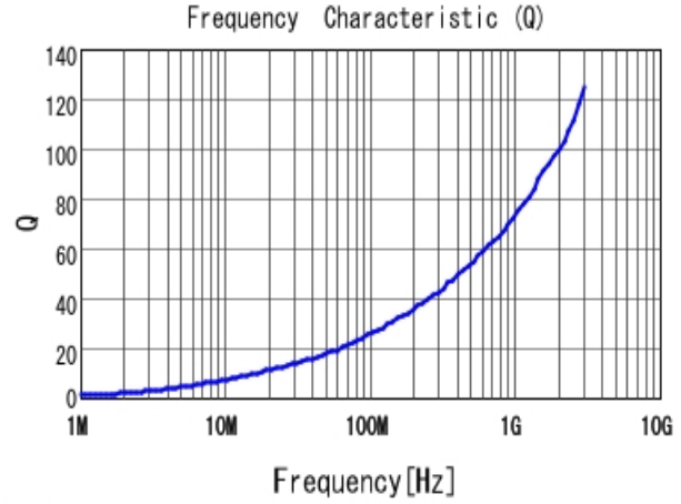
■ LQW15AN3N4D80 Q
