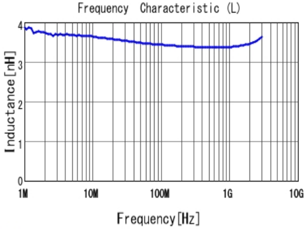
■ LQW15AN3N4D80 L
