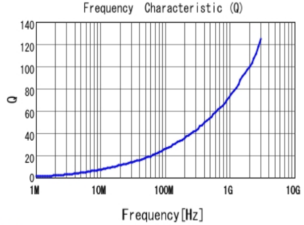
■ LQW15AN3N4B80 Q
