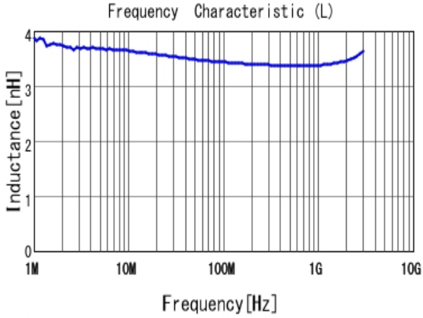
■ LQW15AN3N4B80 L
