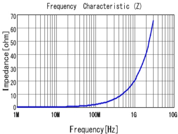
■ LQW15AN3N3G80 |Z|
