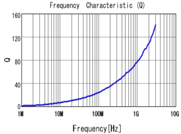
■ LQW15AN3N3G80 Q
