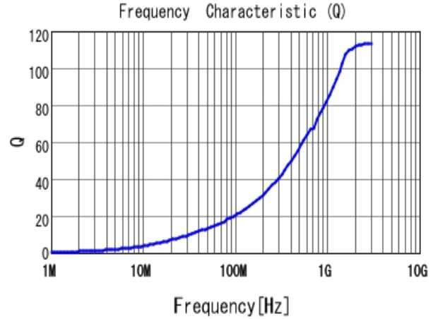
■ LQW15AN3N0G80 Q
