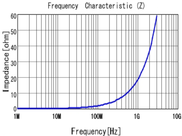
■ LQW15AN3N0G80 |Z|
