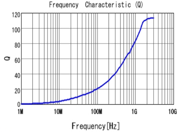
■ LQW15AN3N0D80 Q
