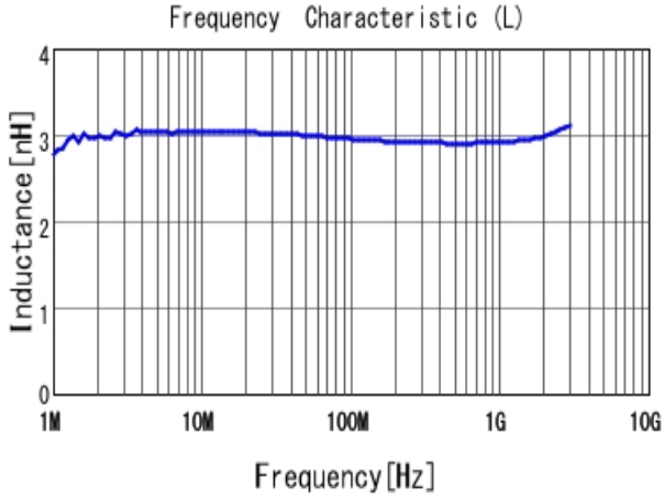
■ LQW15AN3N0D80 L
