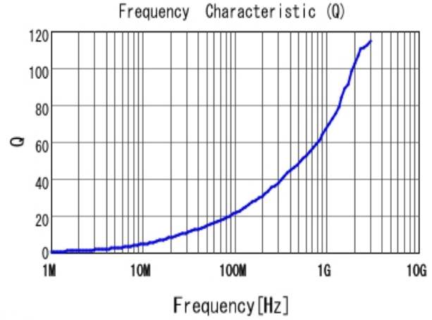
■ LQW15AN2N7G80 Q
