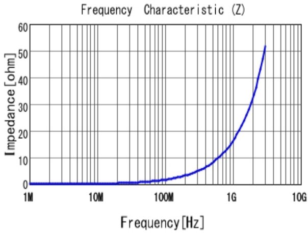
■ LQW15AN2N7G80 |Z|
