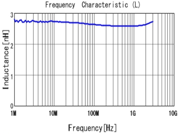
■ LQW15AN2N7G80 L
