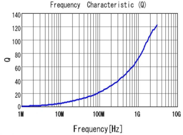
■ LQW15AN2N6B80 Q
