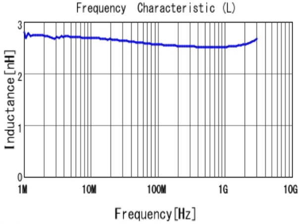
■ LQW15AN2N6B80 L
