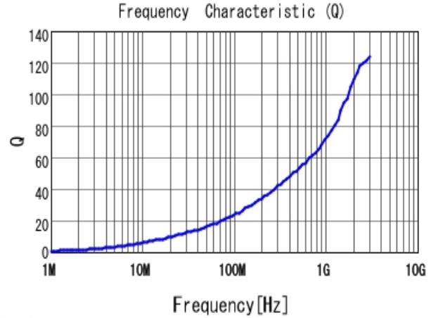
■ LQW15AN2N5G80 Q
