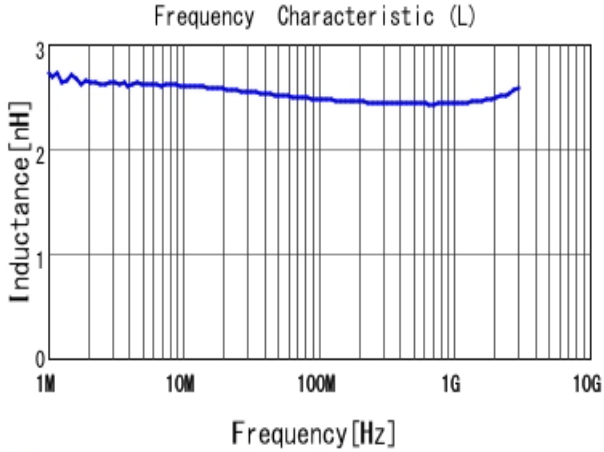
■ LQW15AN2N5G80 L
