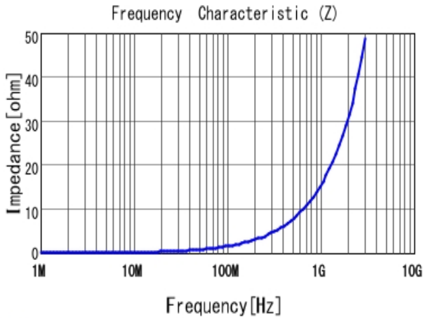
■ LQW15AN2N5D80 |Z|
