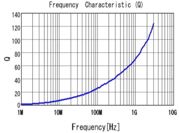
■ LQW15AN2N4D80 Q
