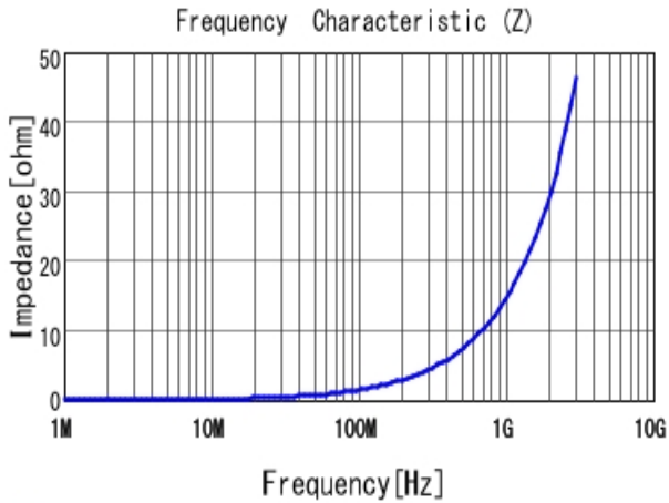
■ LQW15AN2N4D80 |Z|
