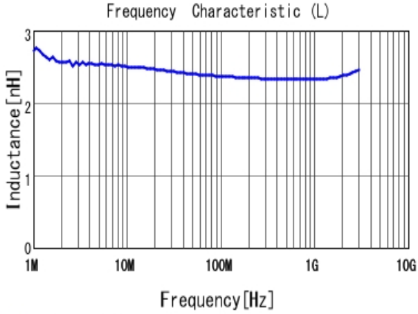
■ LQW15AN2N4D80 L
