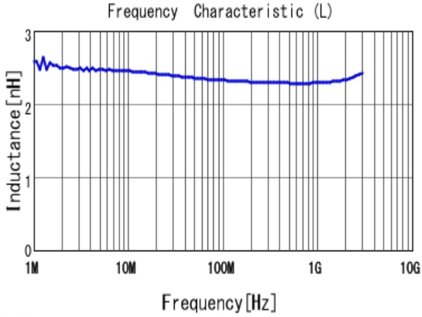
■ LQW15AN2N3B80 L
