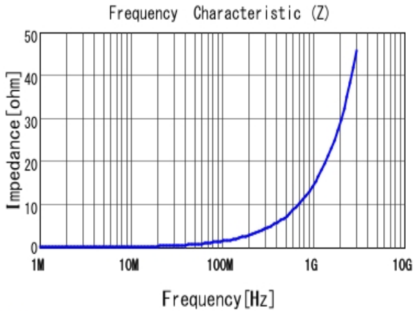
■ LQW15AN2N3B80 |Z|
