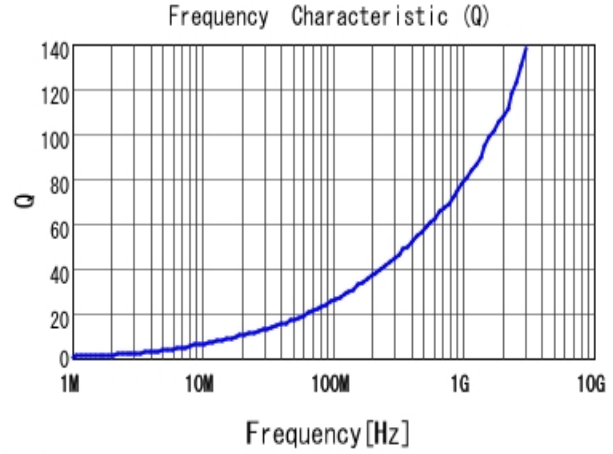
■ LQW15AN2N3B80 Q
