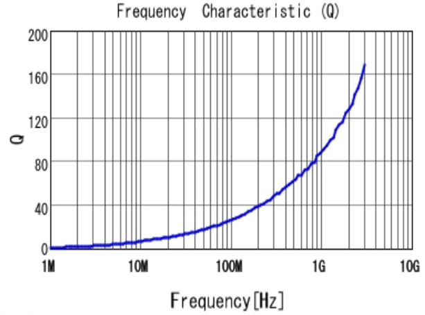
■ LQW15AN2N2D80 Q
