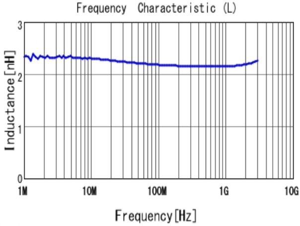
■ LQW15AN2N2D80 L
