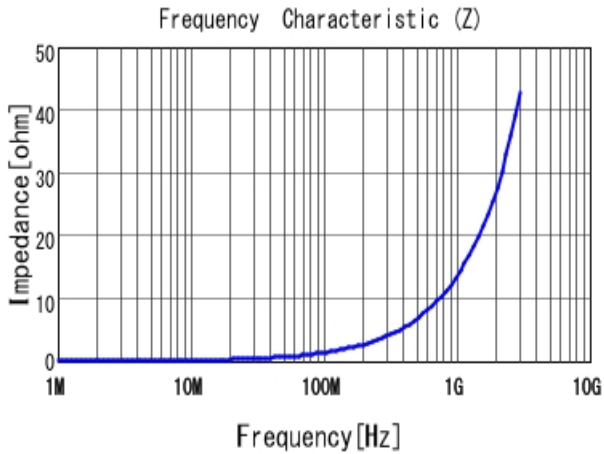
■ LQW15AN2N2D80 |Z|
