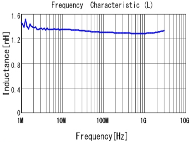
■ LQW15AN1N3D80 L
