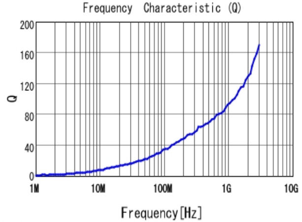
■ LQW15AN1N3D80 Q
