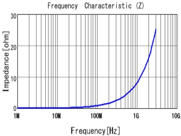
■ LQW15AN1N3D80 |Z|
