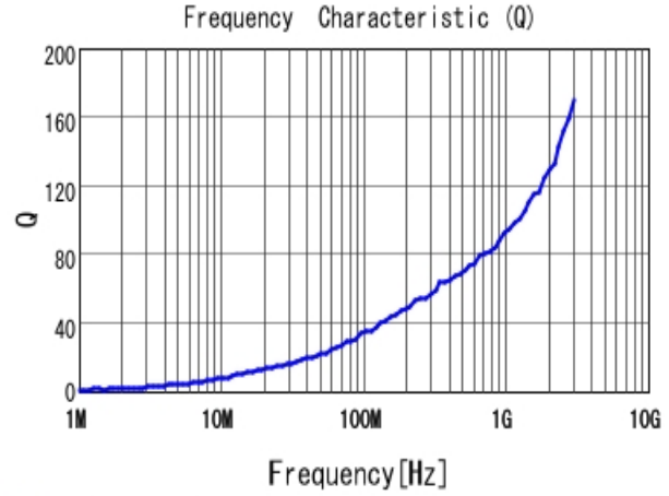
■ LQW15AN1N3C80 Q
