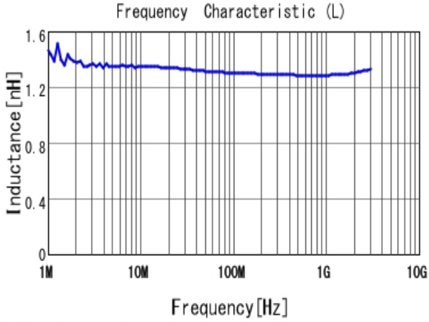
■ LQW15AN1N3C80 L
