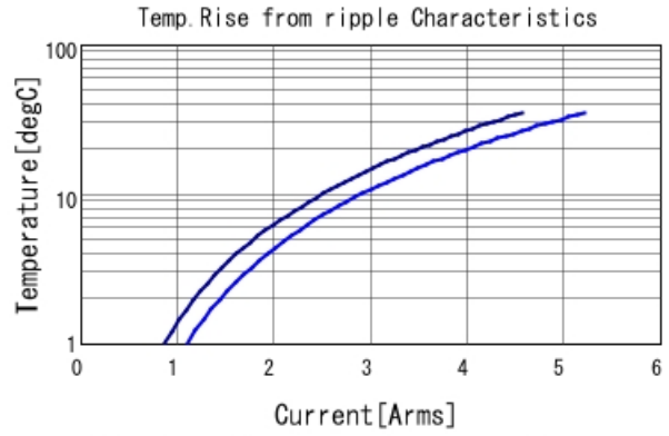
GRM21BR61H475KE51 Temp. rise — 500kHz — 1MHz
