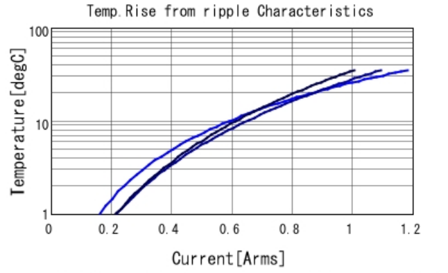
GRM1555C1H820JA01 Temp. rise — 200MHz — 500
