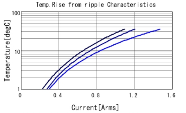
GRM1555C1H560JA01 Temp. rise — 200MHz — 500
