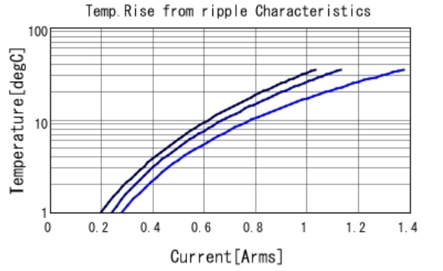
GRM1555C1H510JA01 Temp. rise — 200MHz — 500
