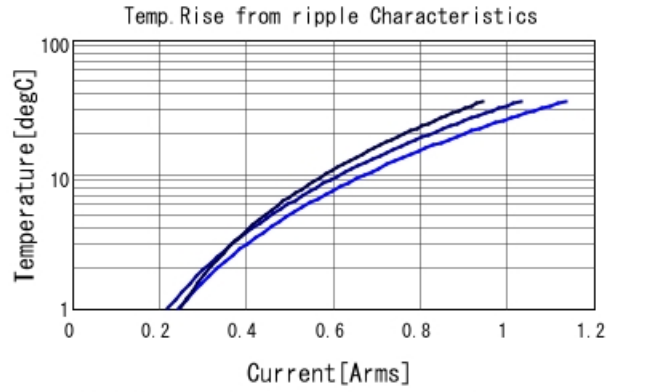
GRM1555C1H430JA01 Temp. rise — 500MHz — 700I
