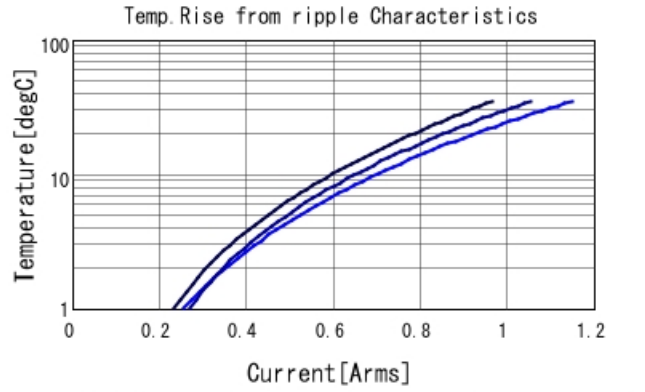
GRM1555C1H390JA01 Temp. rise — 500MHz — 700I
